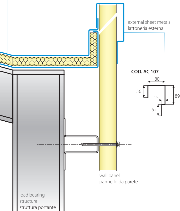
gasket guarnizione
